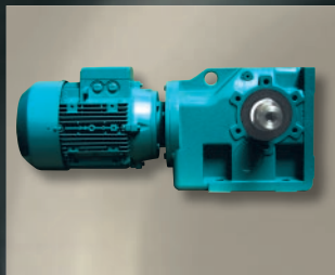
↑ KTM – kuželové převodovky KTM – конические-цилиндрические редукторы Velikost/Размер 3–7 P_1 = 0,37 - 15 \text{ kW/kBm} M_k 100 - 2500 \text{ Nm/Hm}
